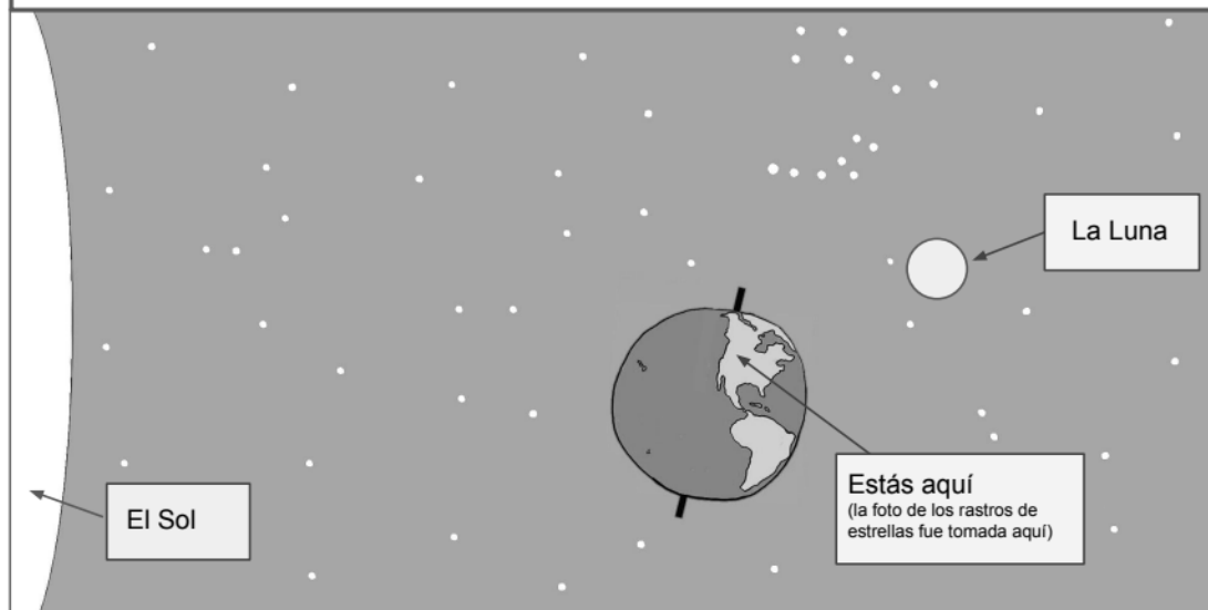
Vista de la Tierra desde el espacio ( no está a escala )
